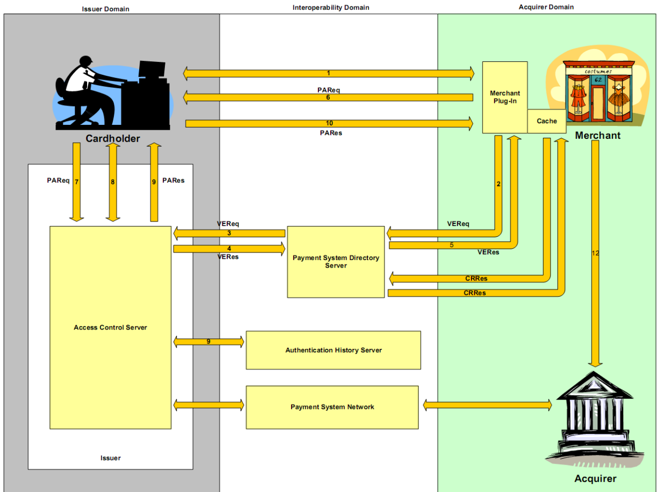
2-Rasm. Internetda to'lov amalga oshirishning bosqichlarga bo'lingan uch domenlik sxemasi
