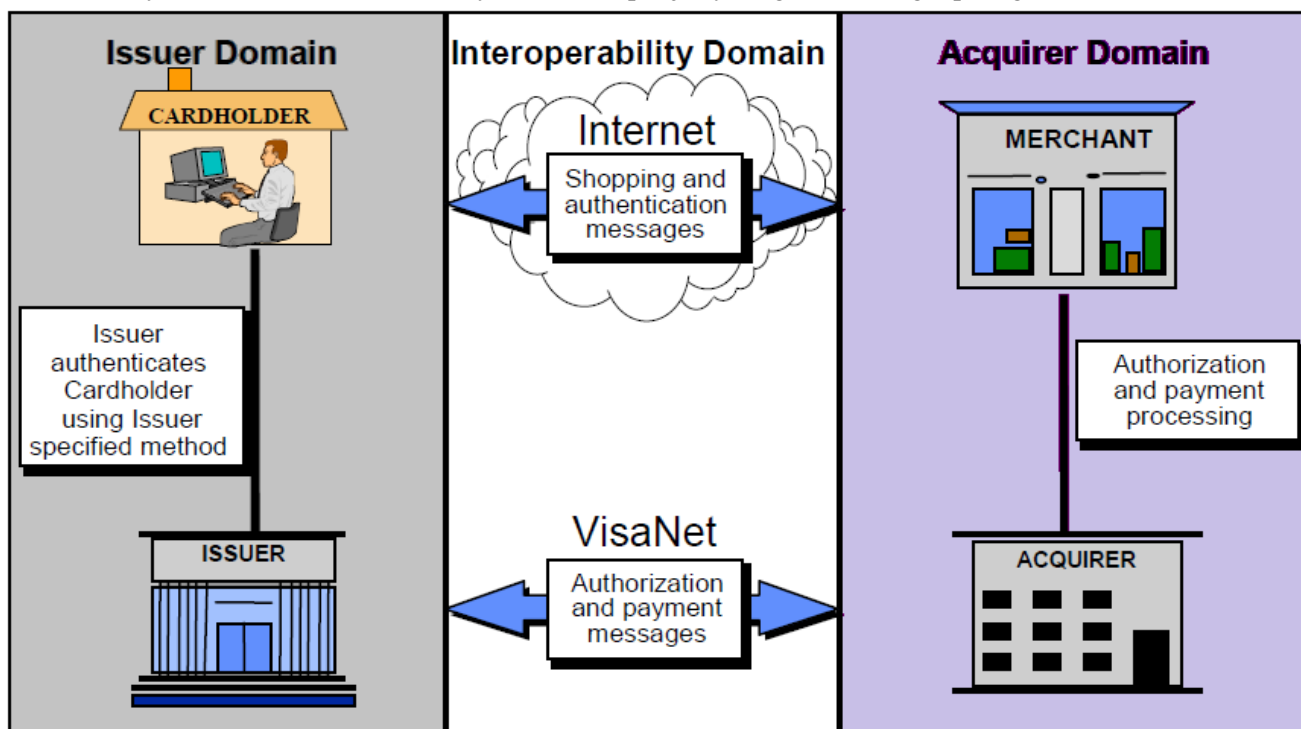
1-Rasm. 3D-Secure protokoli bo'yicha Autentifikatsiyani uch domen modelidan foydalanib joriy qilish.
